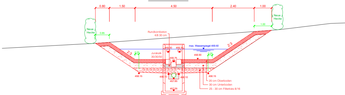
Schnitt B - B
