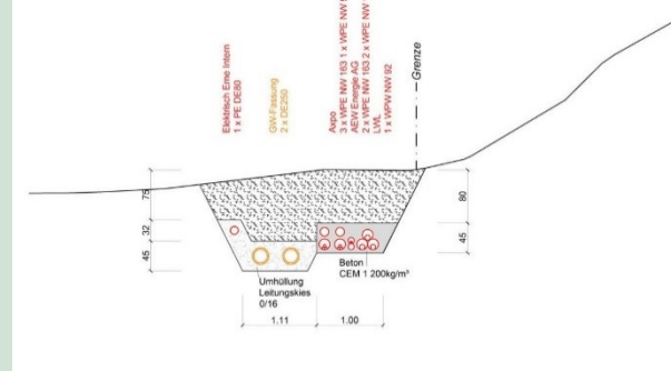
Querschnitt A - A 1 : 50
