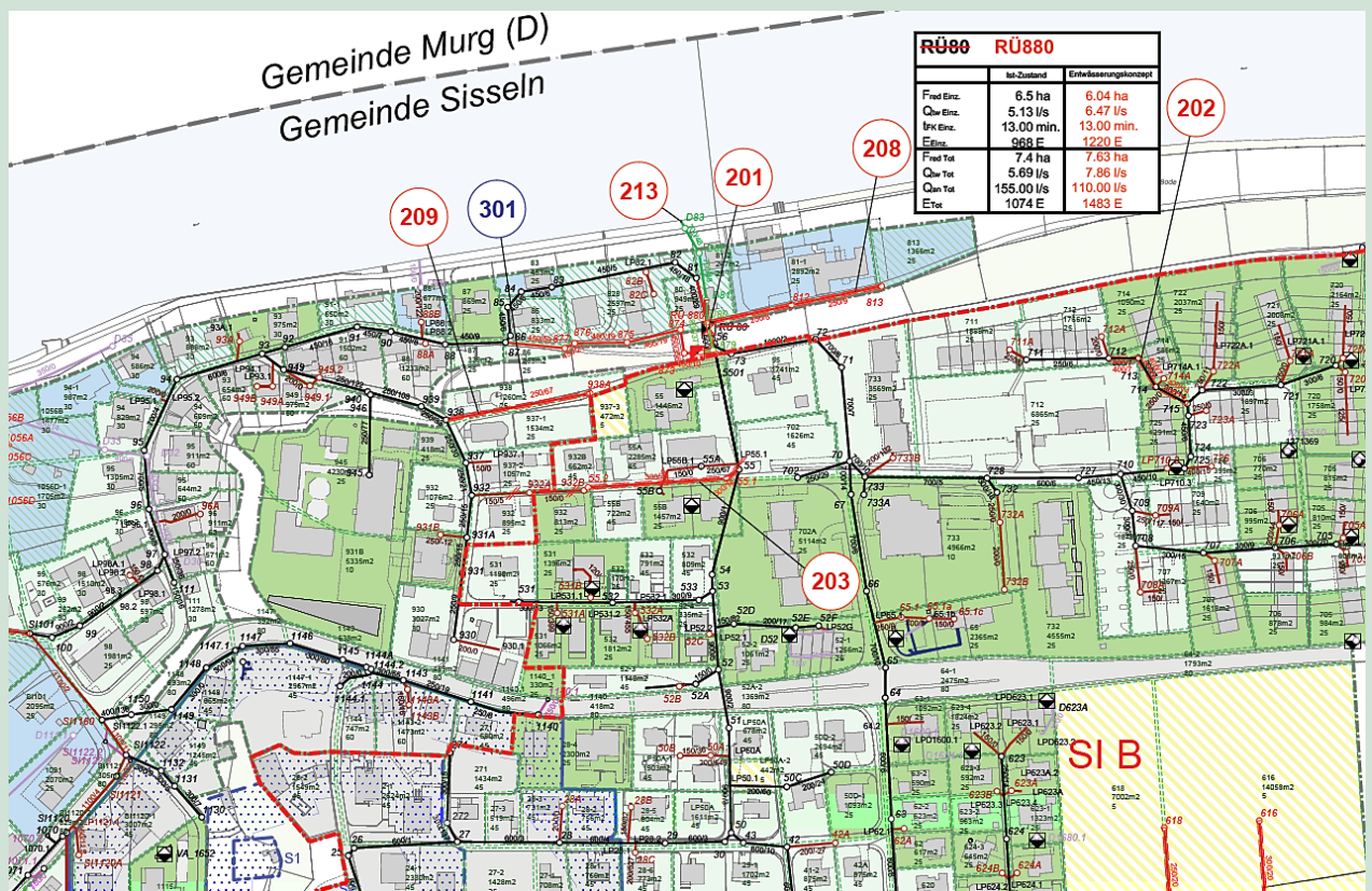
Massnahmenplan mit geplanten Entwässerungssystemen der einzelnen Teileinzugsgebiete innerhalb der Phase 3 des GEP 2. Generation Sisseln.
