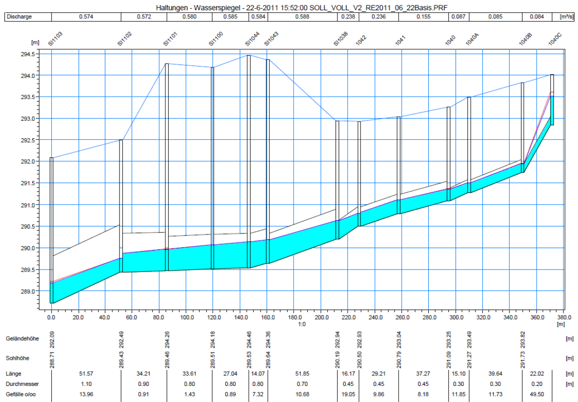
Längenprofil einer überlasteten Leitung. Auszug aus den hydrodynamischen Berechnungen innerhalb der Phase 2 des GEP 2. Generation Sissle.
