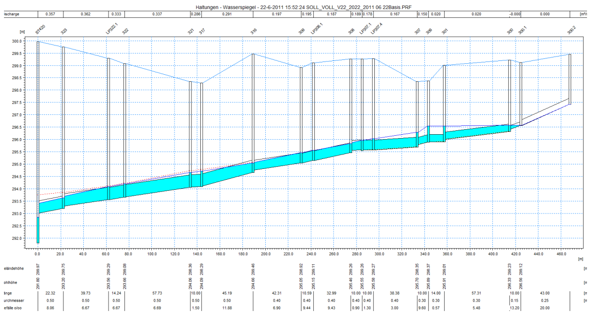
Längenprofil einer überlasteten Leitung. Auszug aus den hydrodynamischen Berechnungen innerhalb der Phase 2 des GEP 2. Generation Stein.
