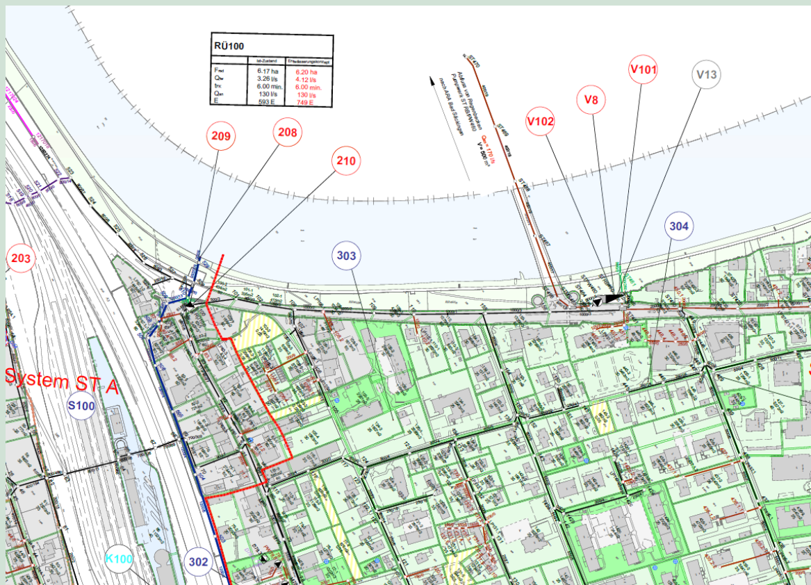
Massnahmenplan mit geplanten Entwässerungssystemen der einzelnen Teileinzugsgebiete innerhalb der Phase 3 des GEP 2. Generation Stein.
